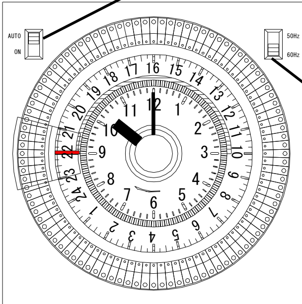
図① 24時間タイマー
