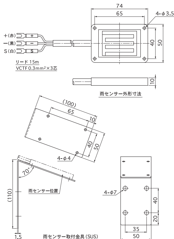
■ 雨センサー・雨センサー取付金具寸法図 (単位:mm)
